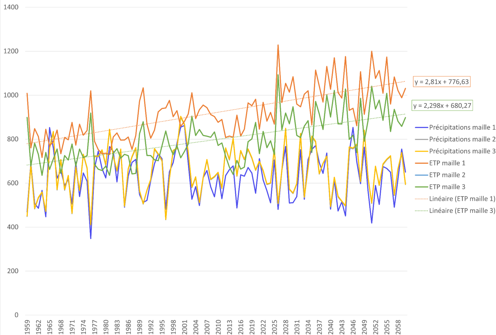
Comparaison précipitations et ETP pour 3 mailles pour la succession 1, sol nu
