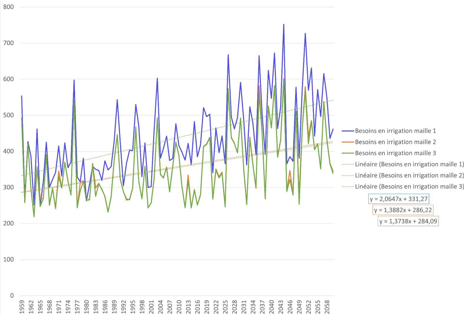
Besoins en irrigation : test de sensibilité mailles pour la succession 1, sol nu
